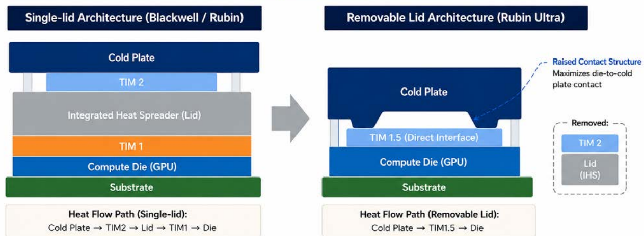
圖 6：Rubin Ultra GPU 世代預計採用可拆卸式上蓋設計，帶動 ASP 持續提升
